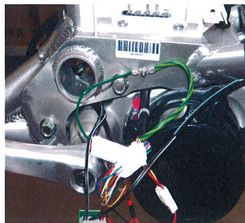
Anschluss Massekabel bei Display 2010/2011
