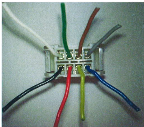
Stecker Displayseitig (Ansicht von oben)
